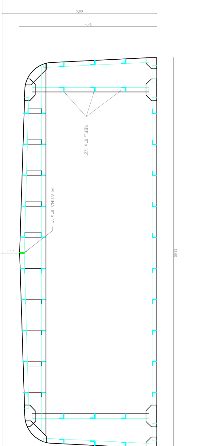
CUADERNA N.º 3
